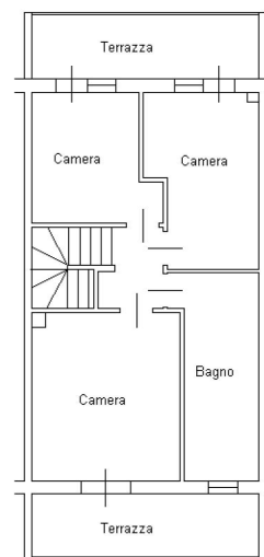
Piano Primo H=270
