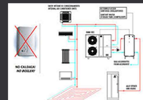
Riscaldamento a pavimento in PdC senza gas
