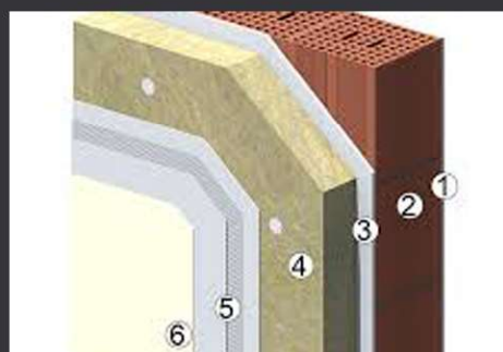
Cappotto lana minerale ignifugo
