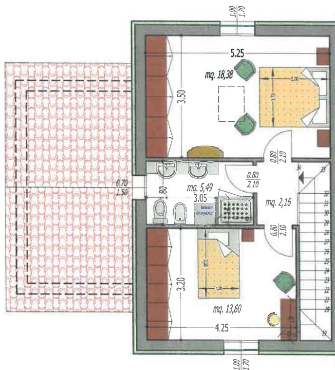
PIANO PRIMO
