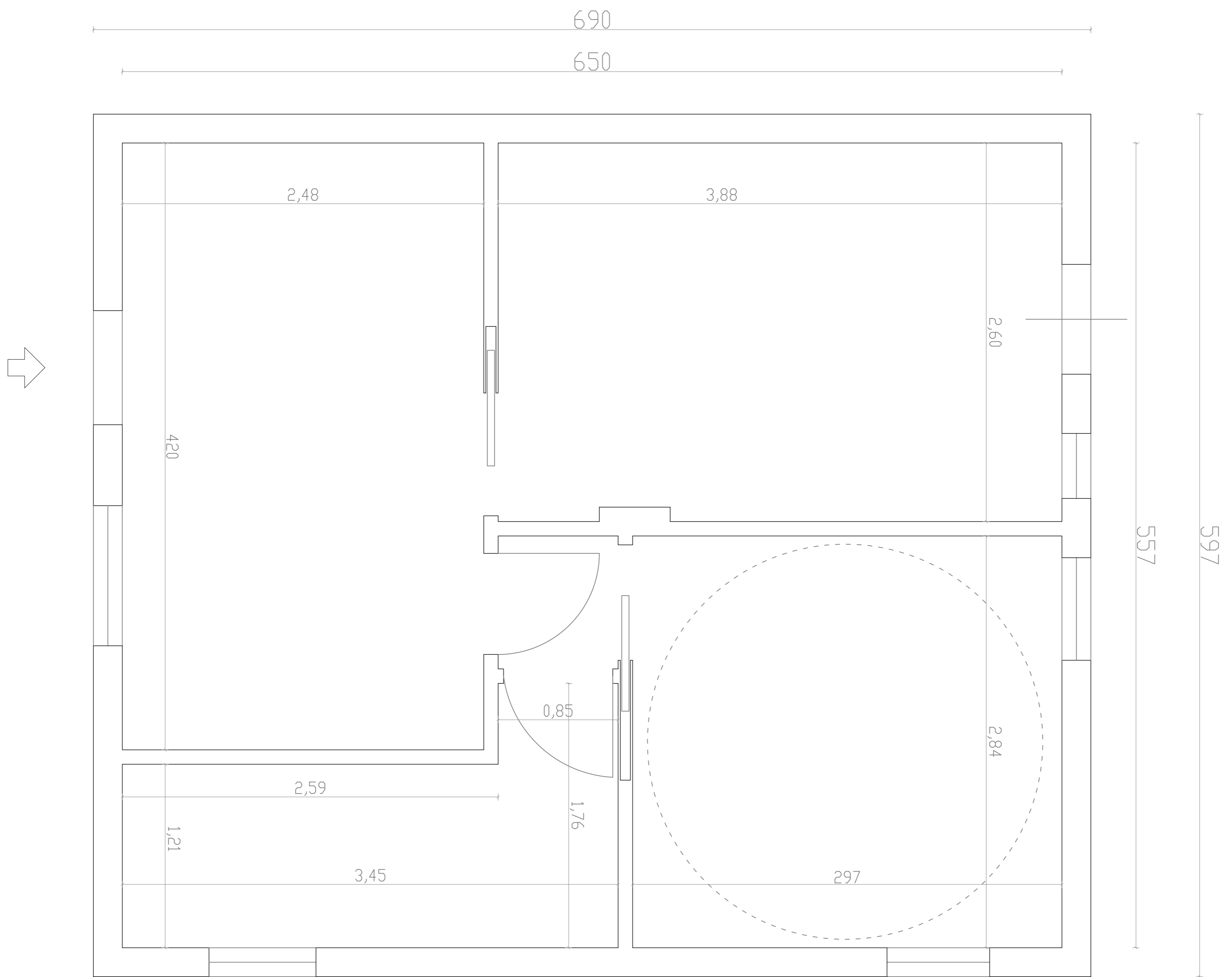
PLANIMETRIA CON LE MISURE DI MASSIMA
