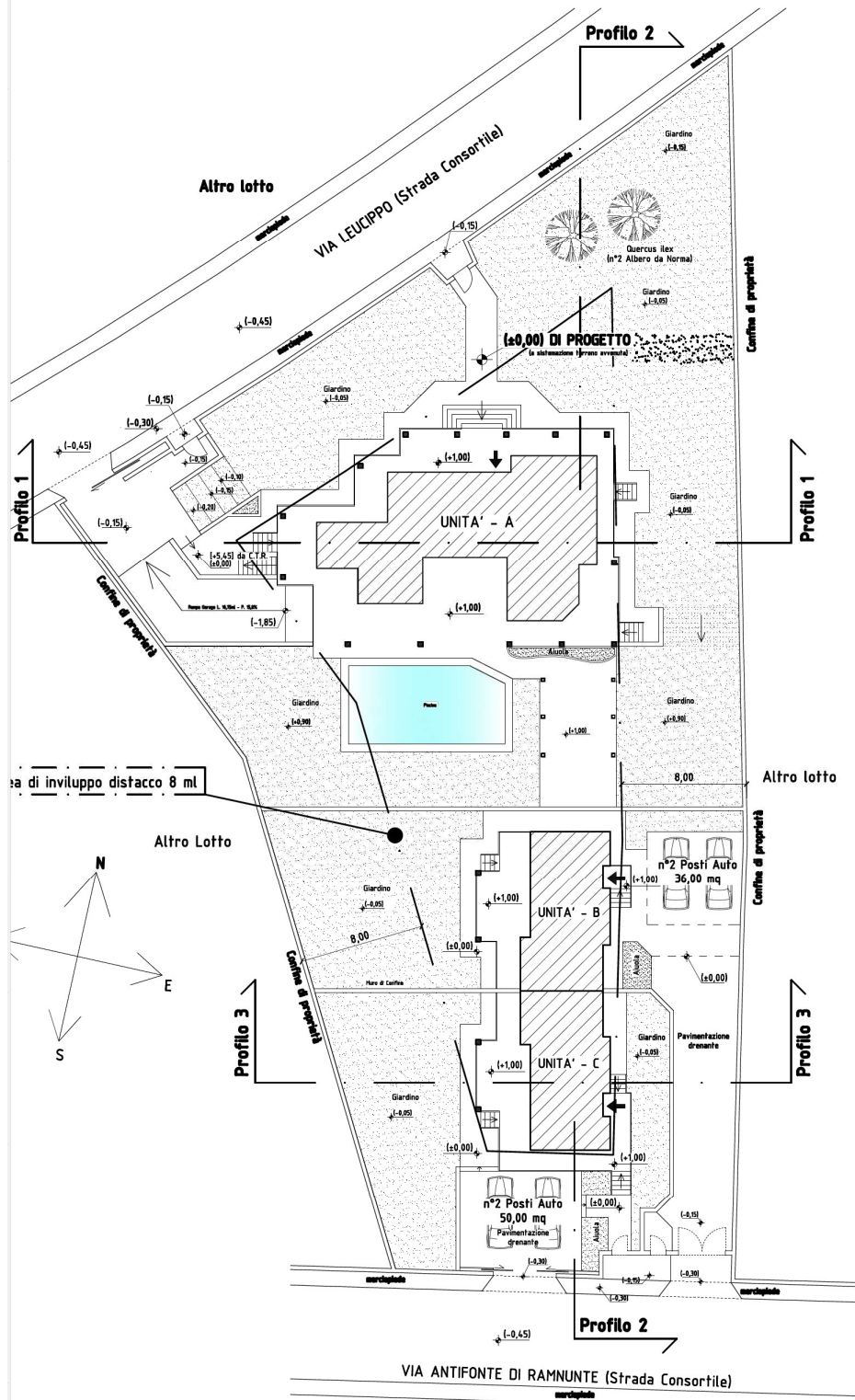
PLANIMETRIA GENERALE - POST OPERAM - Sc. 1:200
