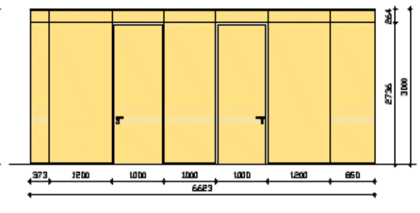
PROSPETTO PARETE DIVISORIA B-B
