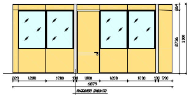
PROSPETTO PARETE DIVISORIA D-D
