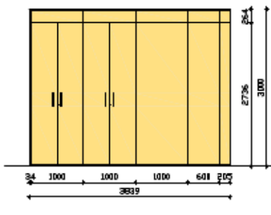
PROSPETTO PARETE ATTREZZATA C-C
