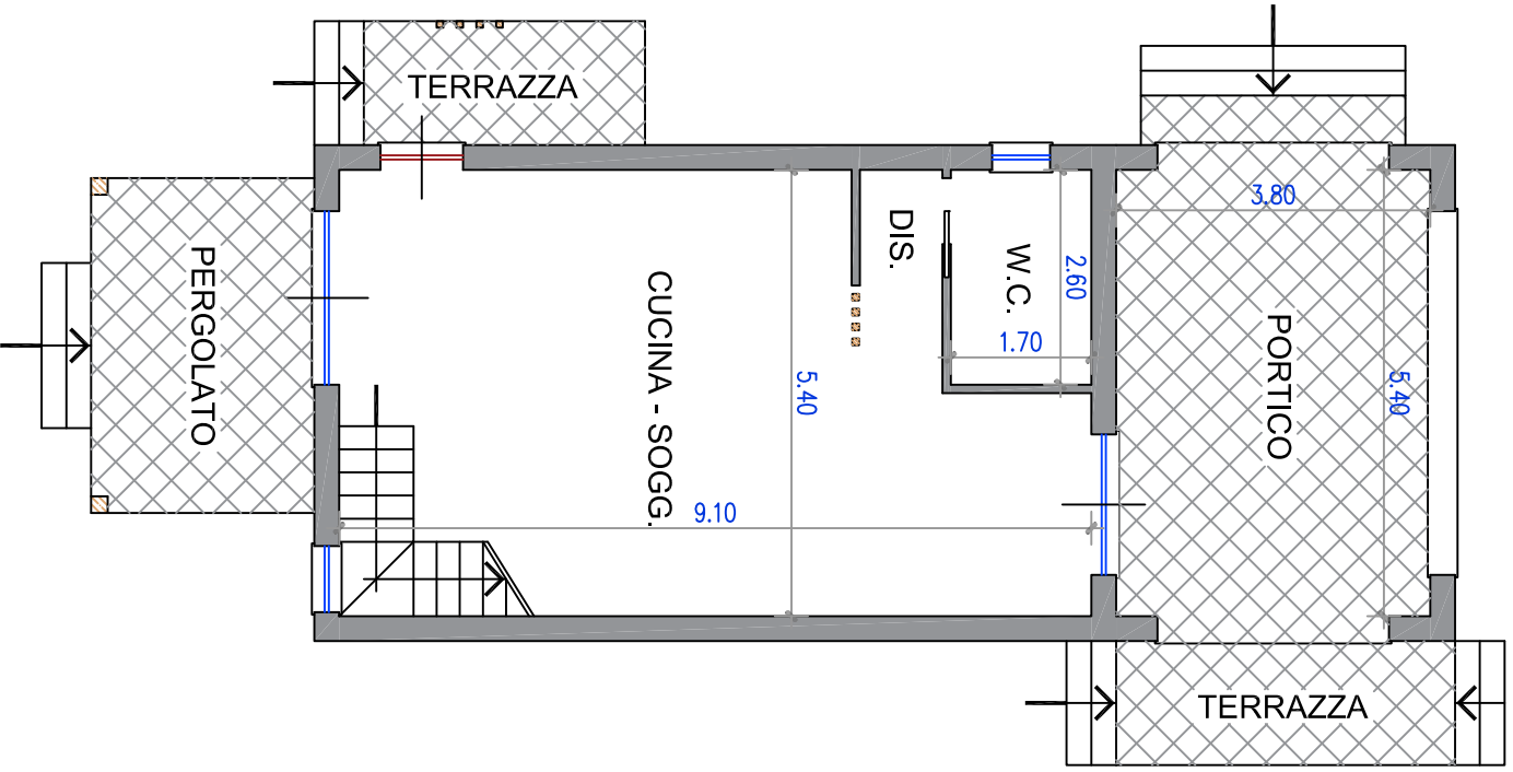
PIANTA PIANO TERRA - Sc. 1:100
