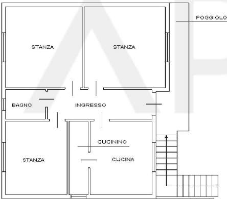
PIANTA PIANO PRIMO H. 3.00
