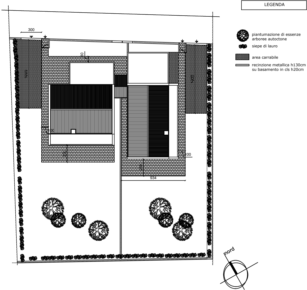
PLANIMETRIA DELLA SISTEMAZIONE ESTERNA
