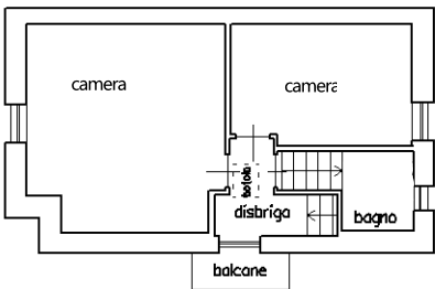
Piano Primo
