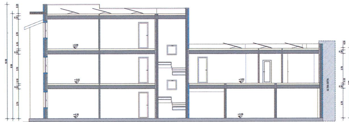
SEZIONE A-A
