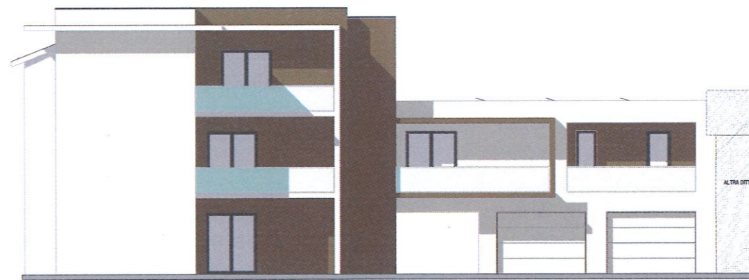
PROSPETTO OVEST
