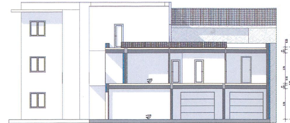
SEZIONE B-B
