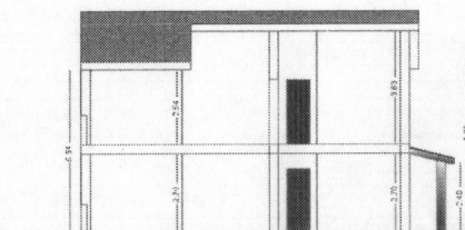
SEZIONE B - B
