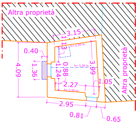
PIANO TERRA - RILIEVO
