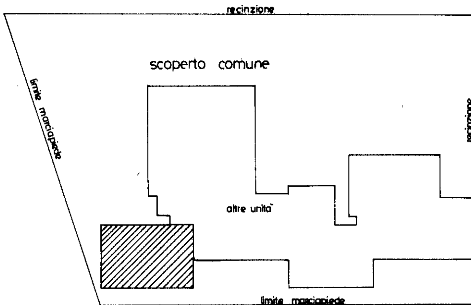
Planimetria 1:500
