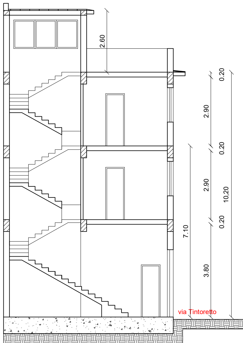
SEZIONE A - B
