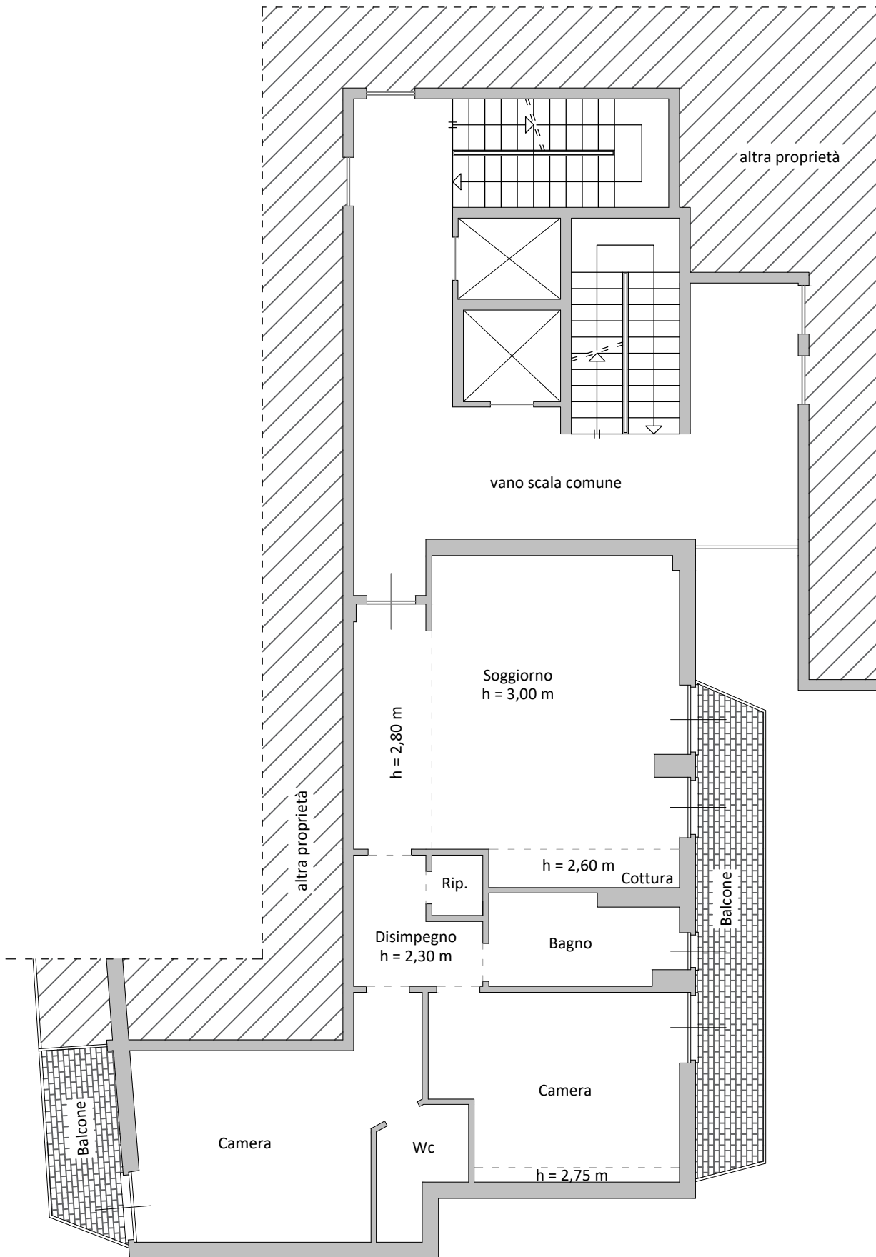
Piano primo STATO DI PROGETTO
