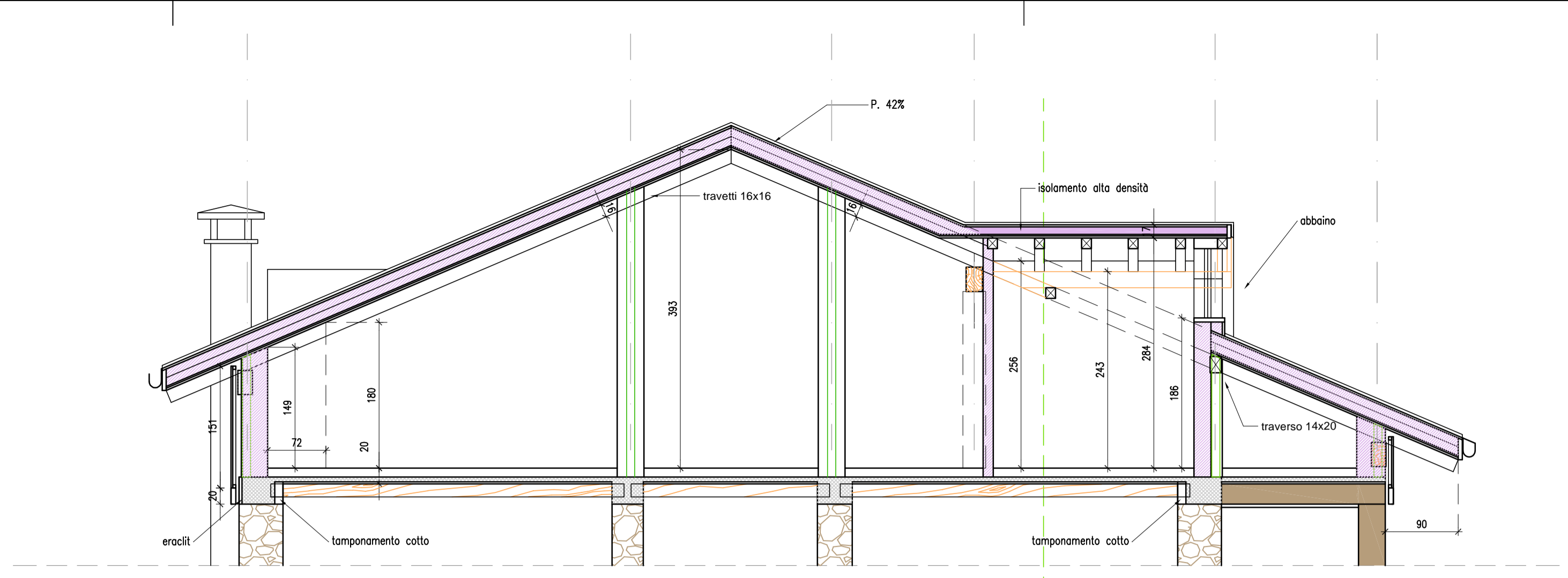
PARTICOLARE ABBAINO
