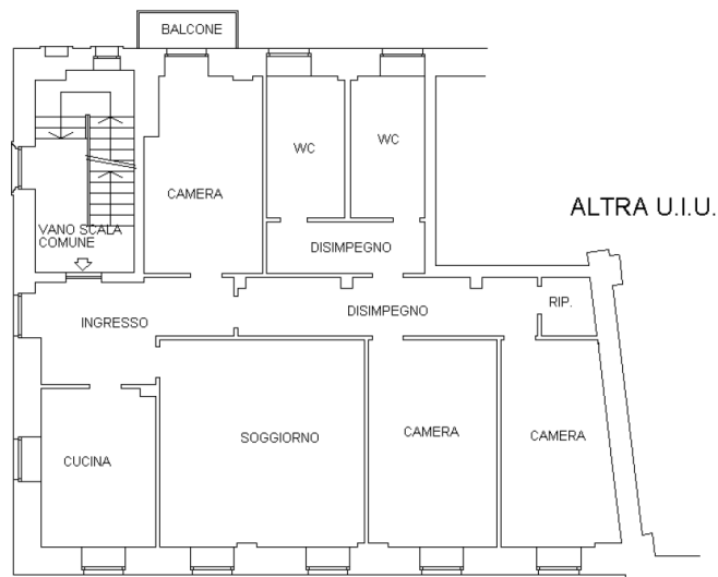
Pianta Piano Secondo – sub. 7 - LOTTO 3
