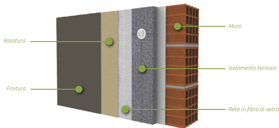
B2 -f _ Isolamento perimetrale a cappotto
