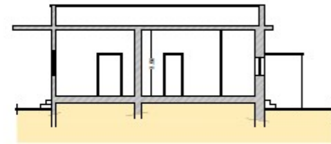
SEZIONE A-A scala 1:100
