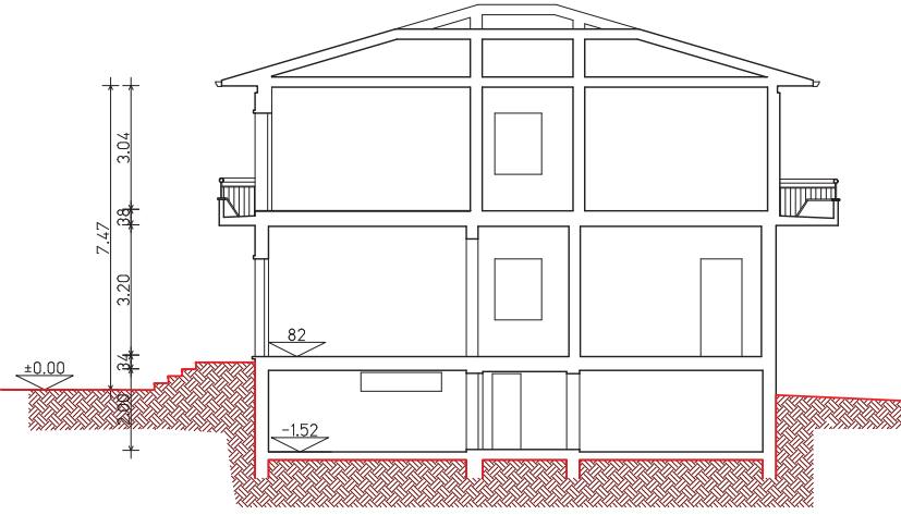
SEZIONE A-B
