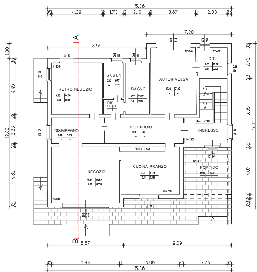
PIANTA PIANO TERRA RIALZATO
