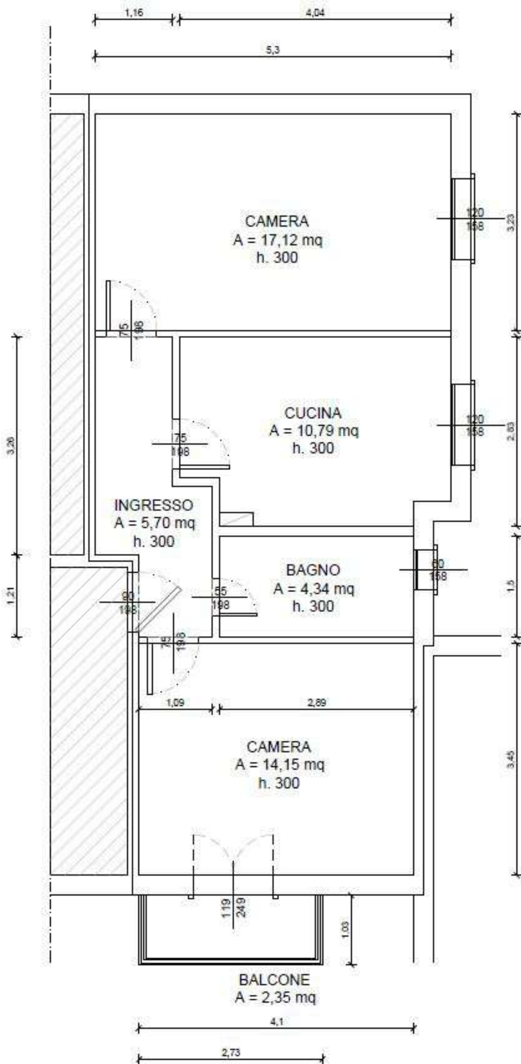
PIANO PRIMO
