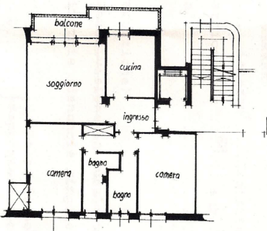
PIANO PRIMO h= 2.99 m
