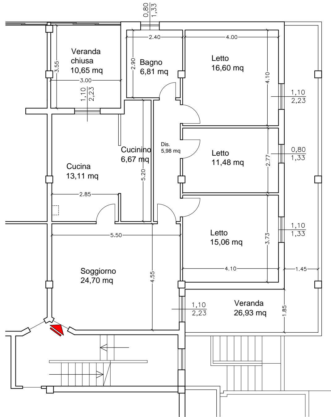
PIANO SECONDO
