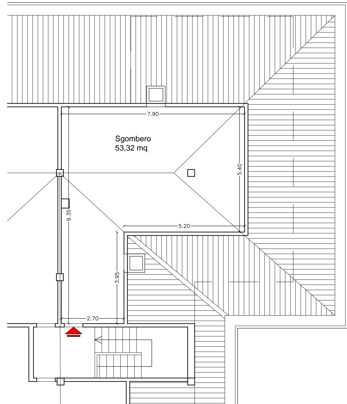
PIANO TERZO
