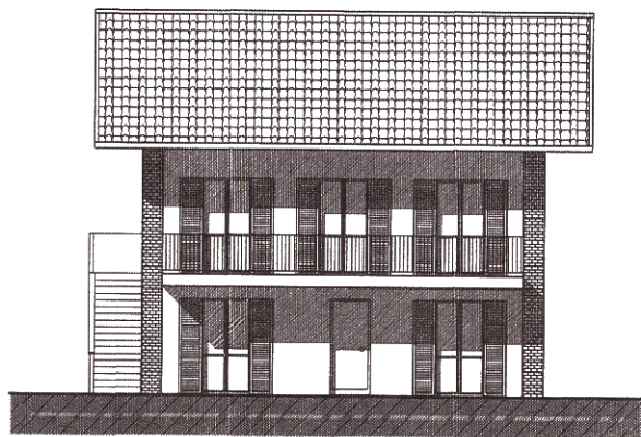
PROSPETTO SUD scala 1:100
