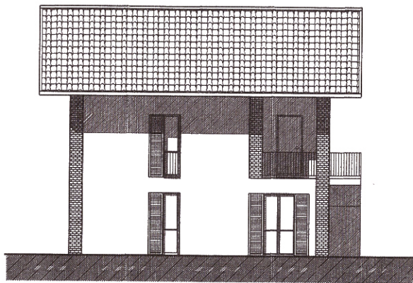
PROSPETTO NORD scala 1:100
