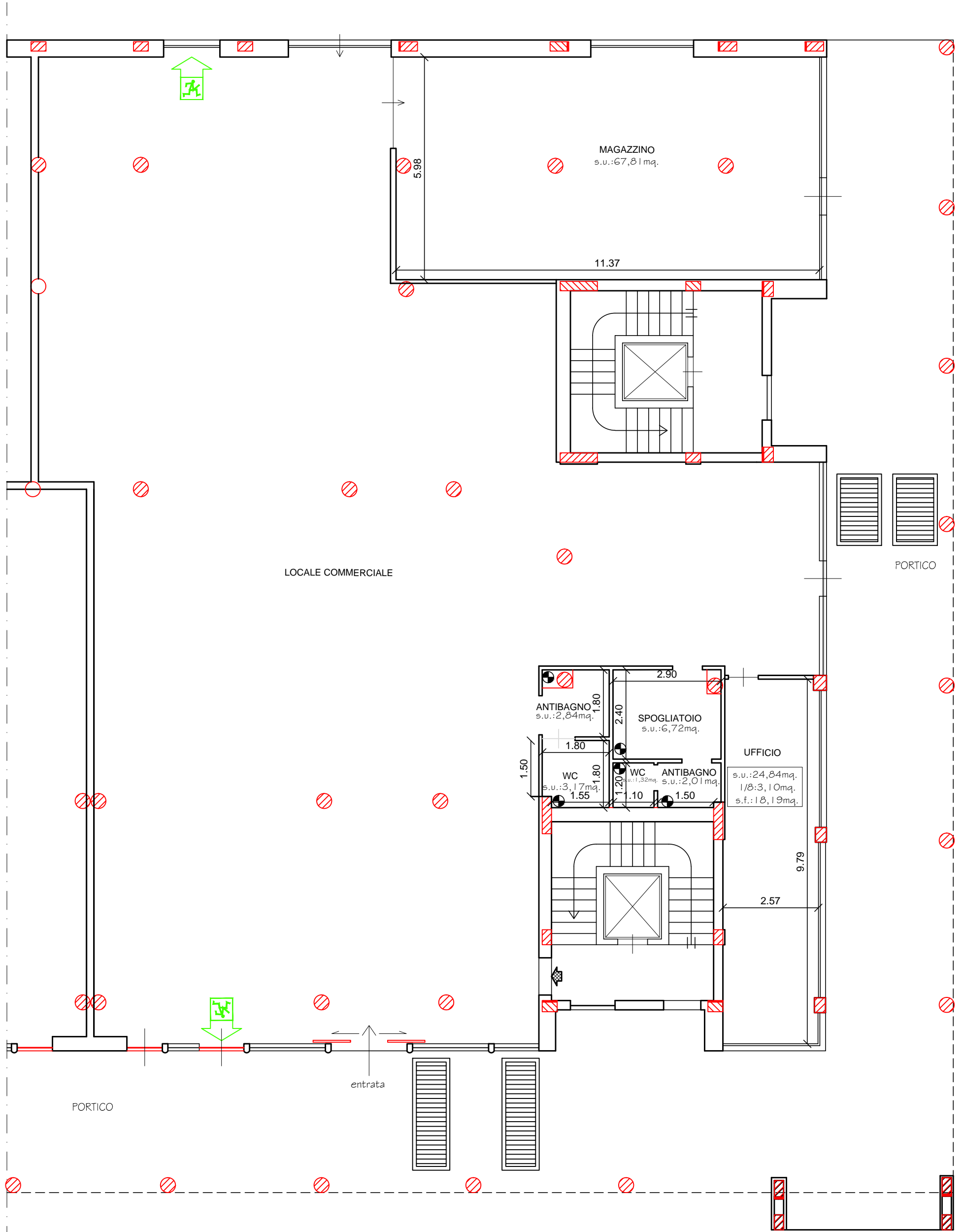
PIANTA PIANO TERRENO
