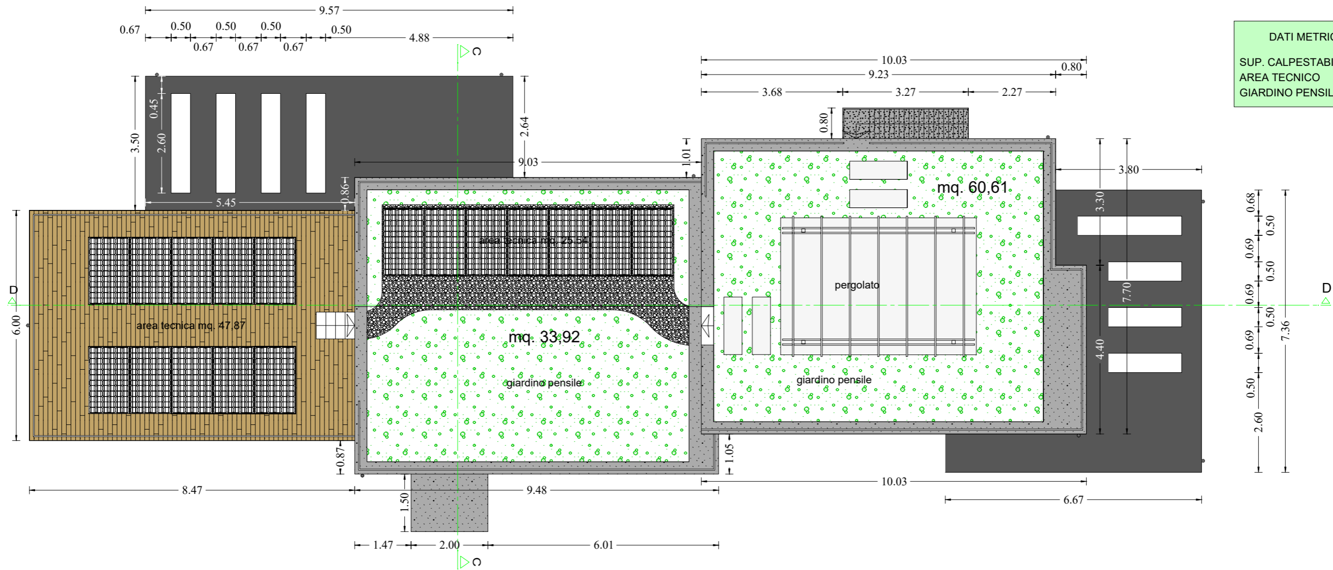
Pianta copertura
