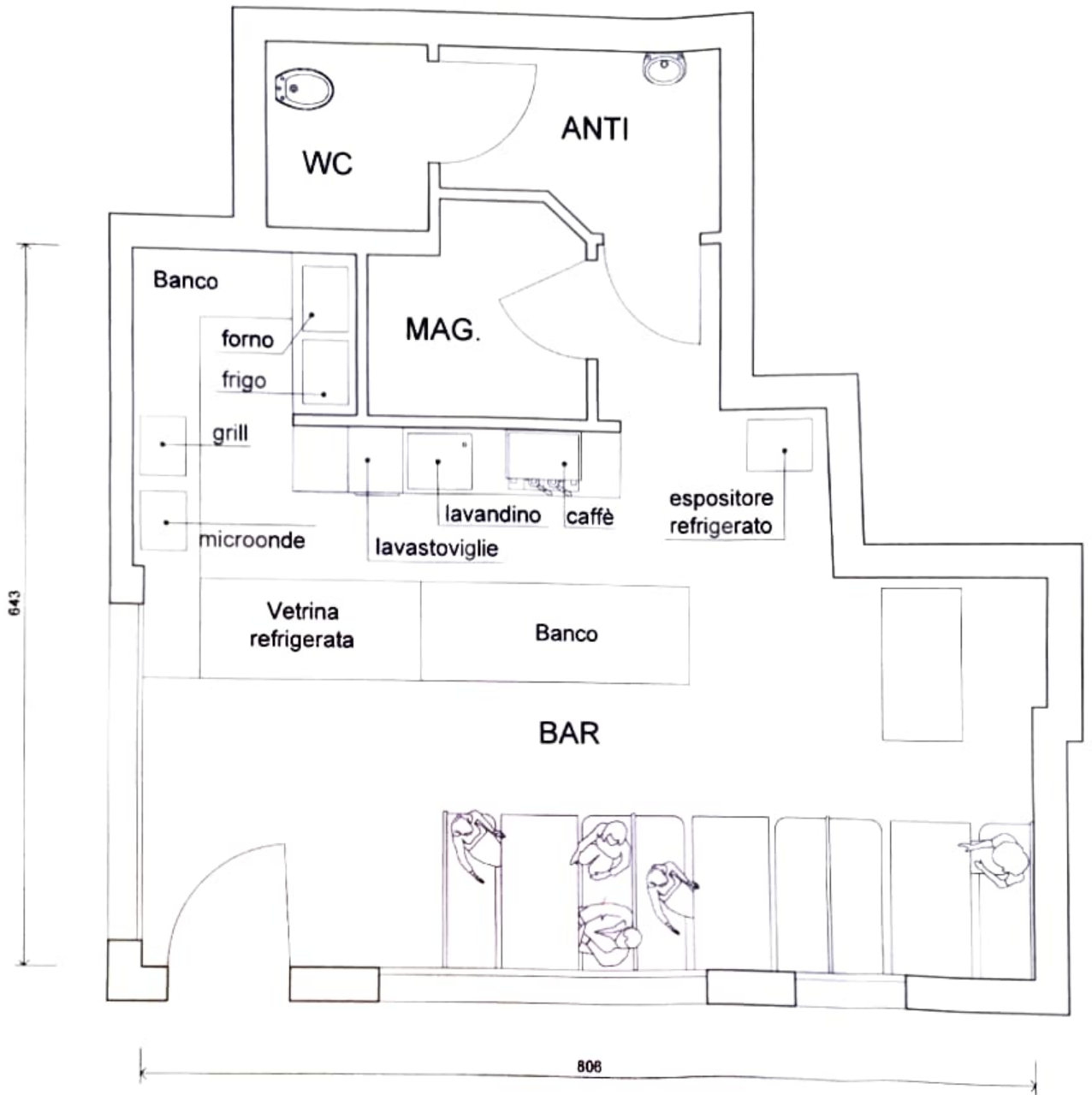
PIANTA PIANO TERRA 1:50
