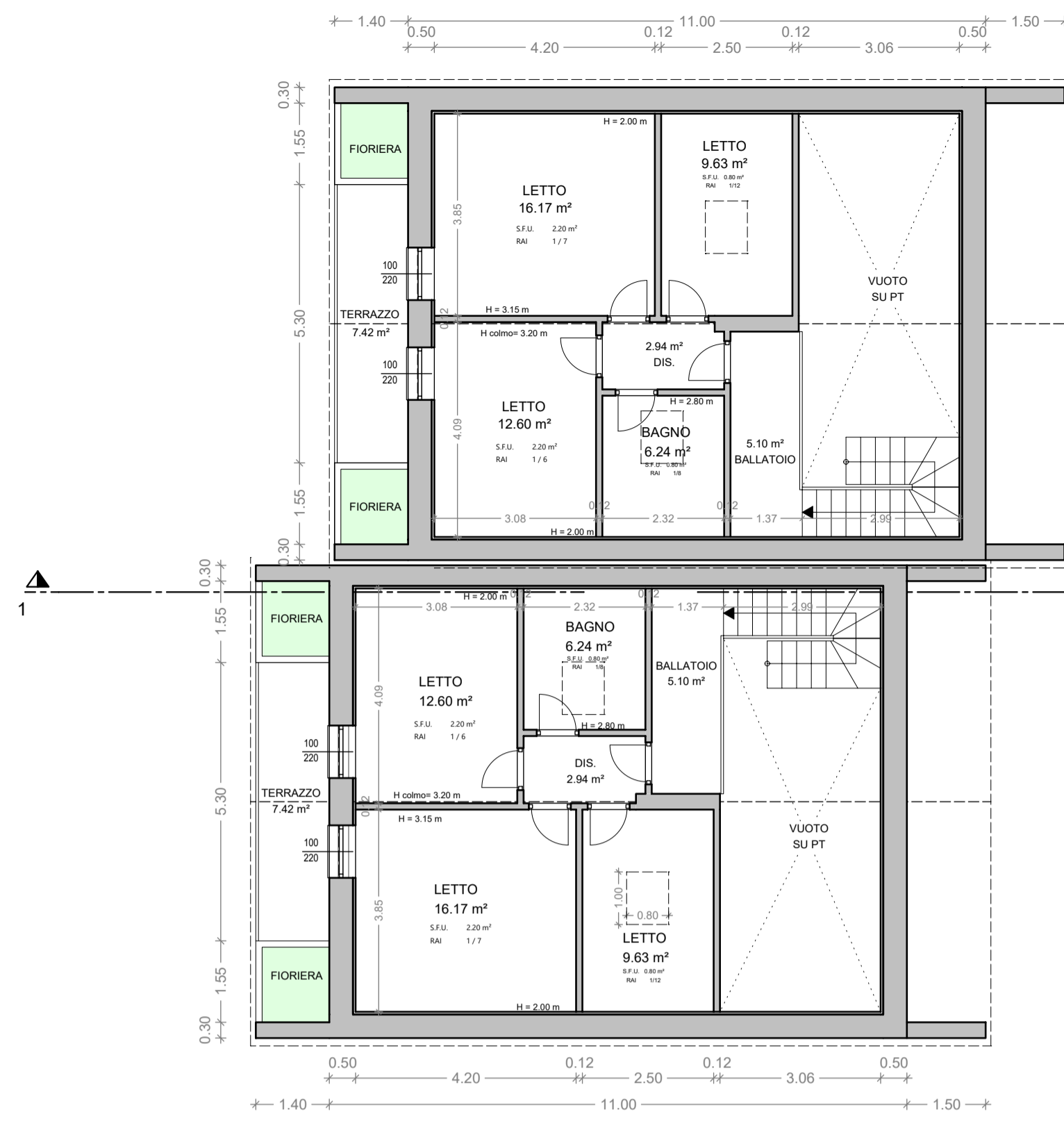
PIANO SECONDO SOTTOTETTO
