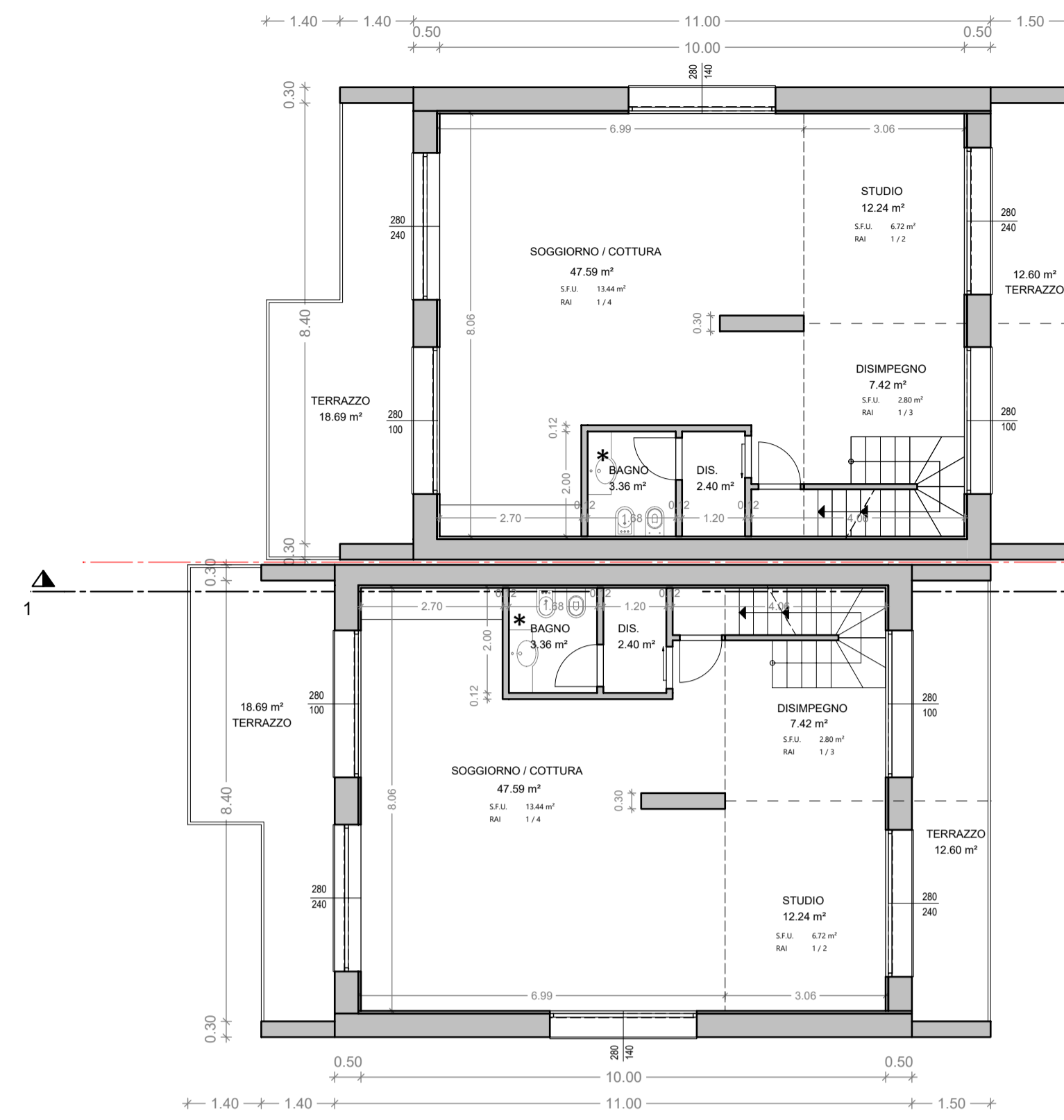
PIANO PRIMO H=2.70 m * LOCALE DOTATO DI ASPIRAZIONE FORZATA
