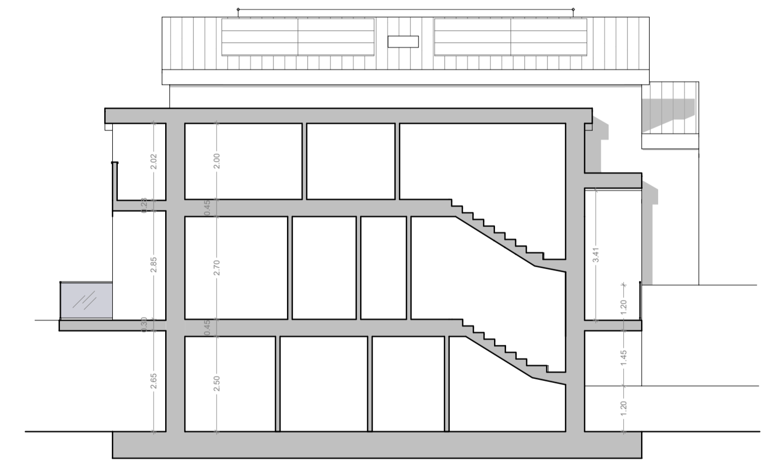
SEZIONE 1-1
