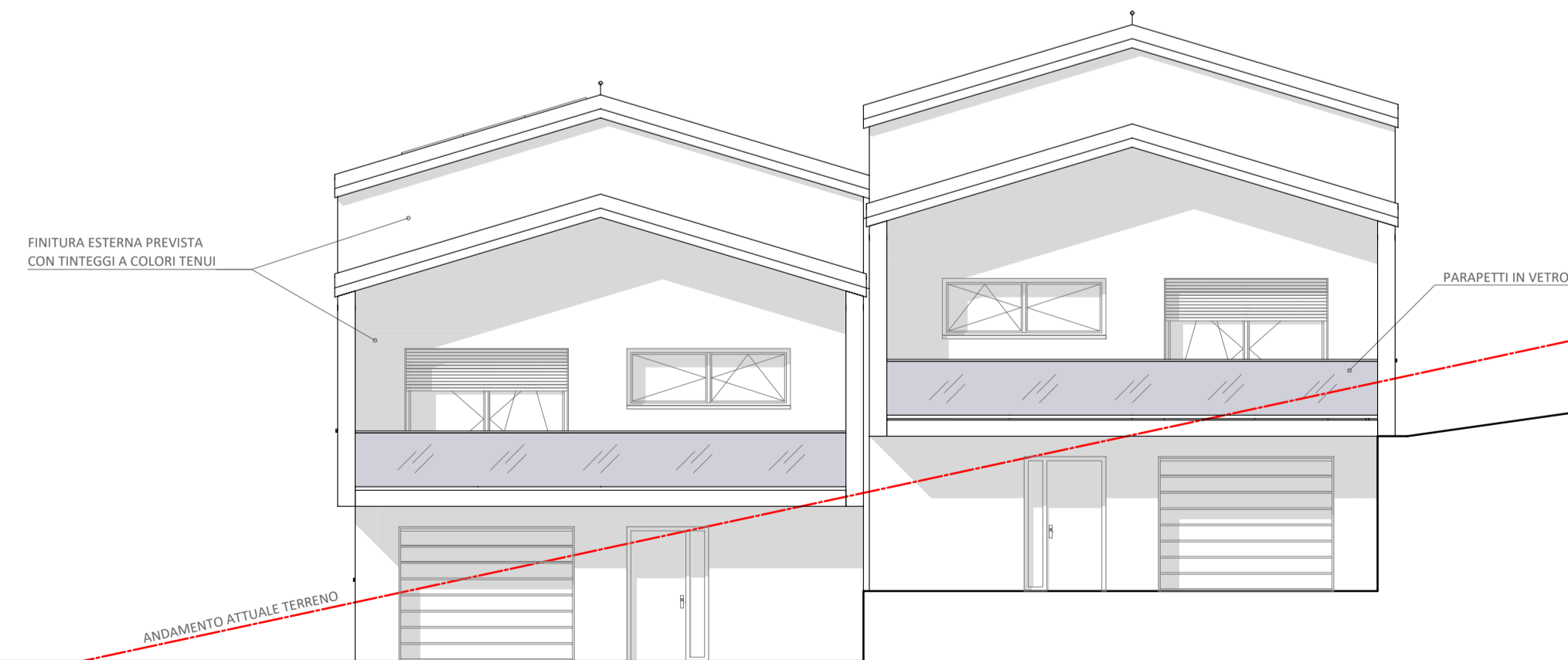
PROSPETTO EST
