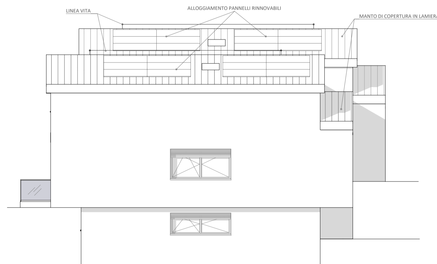
PROSPETTO SUD
