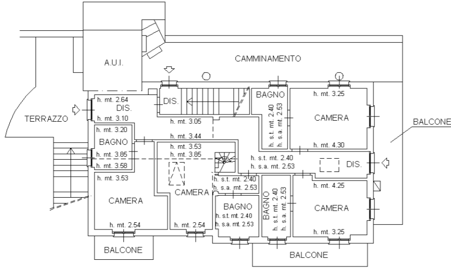
PIANO PRIMO
