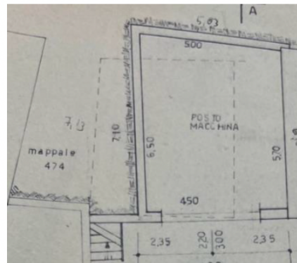
piano primo h = mt. 2,45
