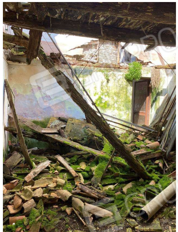
vista interna della stanza ingresso al piano terra con primo solaio in legno crollato
