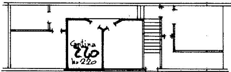
PIANO SOTTERRANEO SCALA 1:200
