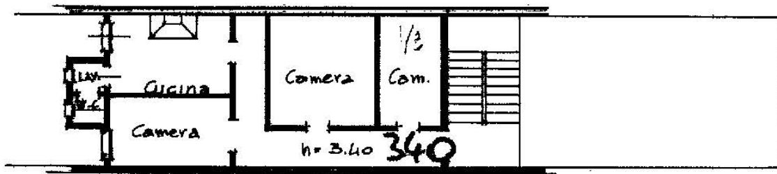
PIANO 1° SCALA 1:200
