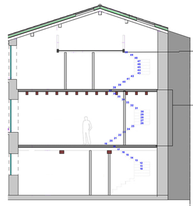
REZIONE A-A'
