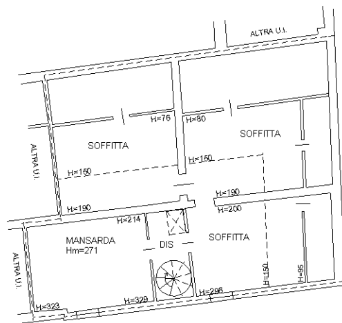
PIANO TERZO
