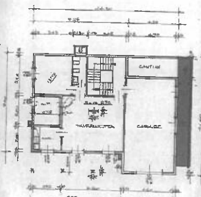
PIANTA PIANO SEMIBASAMENTO SCALE SCALA 1:1000
