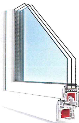
Serramento T-Passive Classic - triplo vetro, 7 camere
