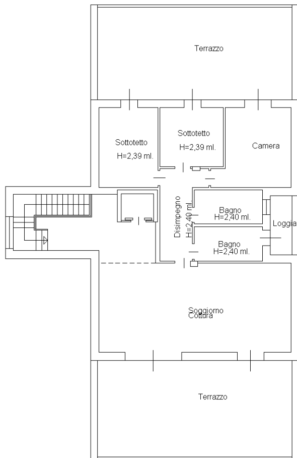
PIANO SECONDO H=2,70 ml.
