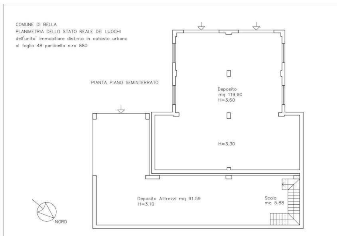
Planimetri dello stato reale dei luoghi Fg 48 particella 880 piano seminterrato (Allegato n. 10)
