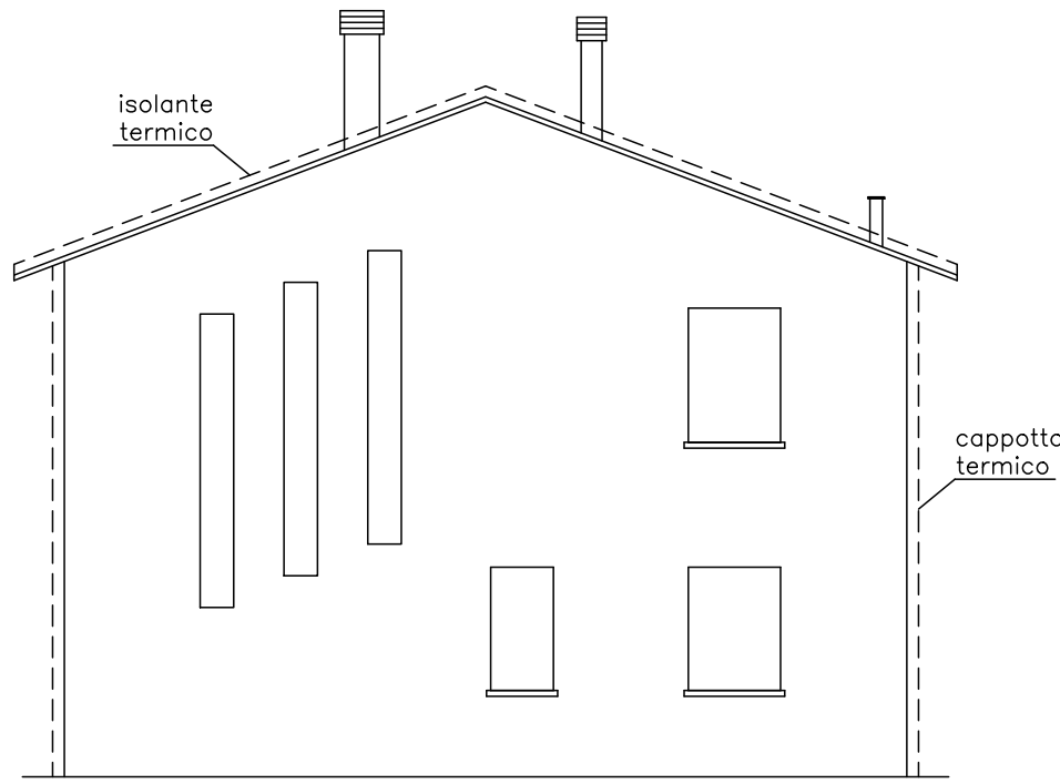
PROSPETTO SUD-EST
