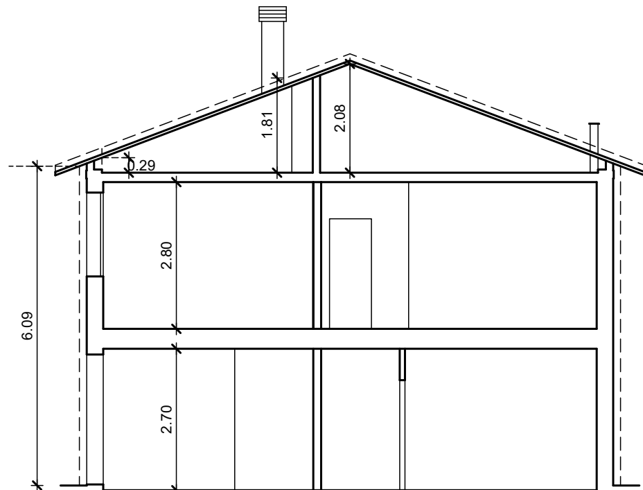
SEZIONE A-A
