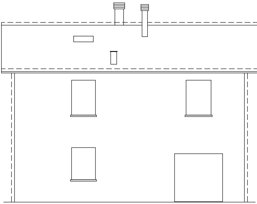
PROSPETTO NORD-EST
