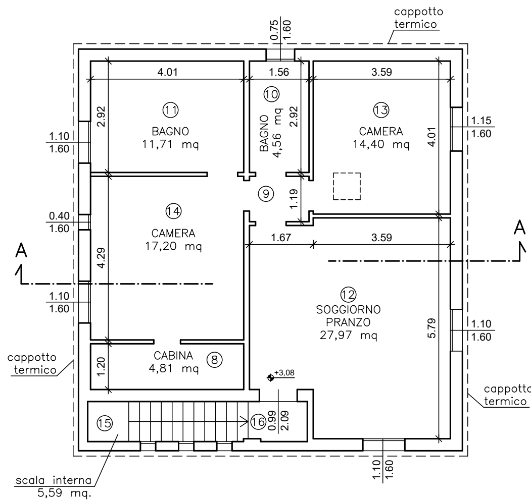
PIANO PRIMO
