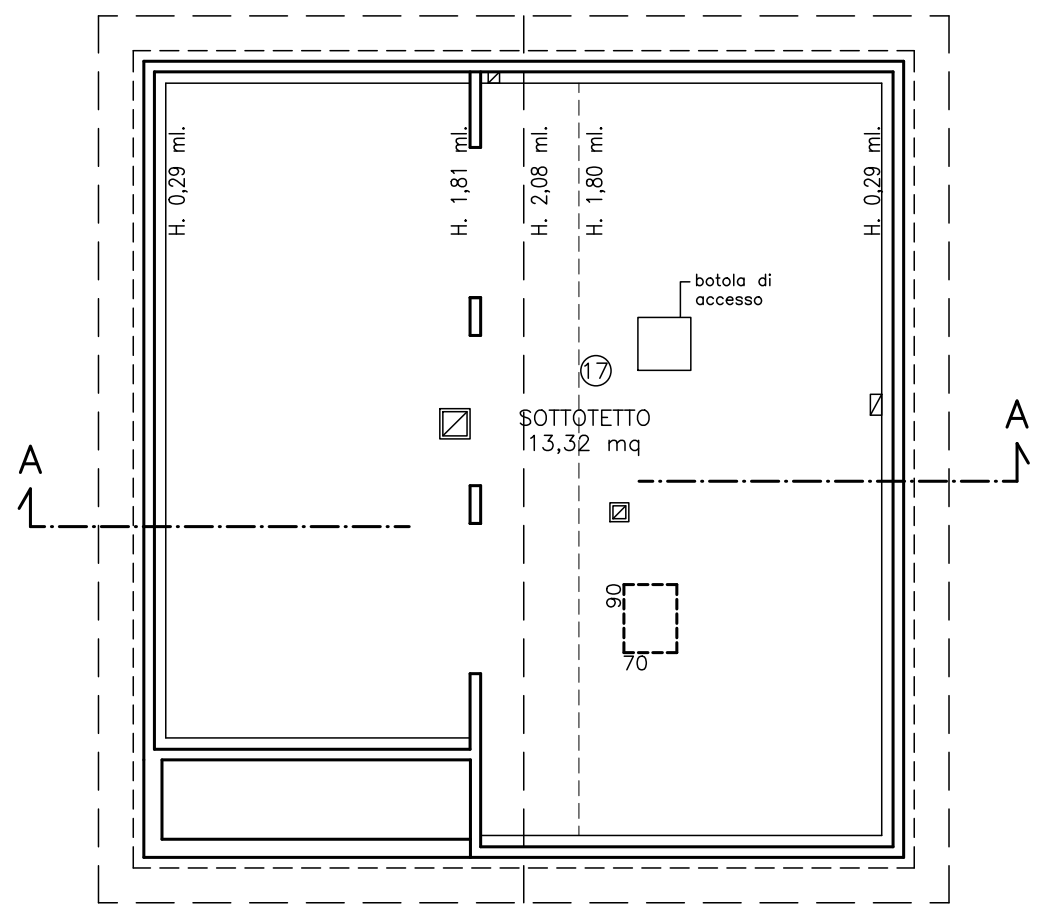
PIANO SOTTOTETTO
