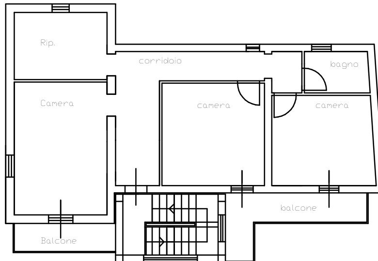
PIANTA PIANO SECONDO H. 2.80
