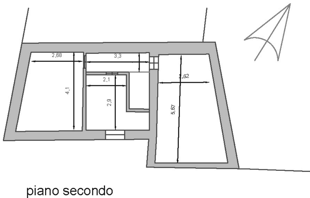
Figura 1 – Corpo A- Abitazione con magazzino – rilievo stato di fatto
