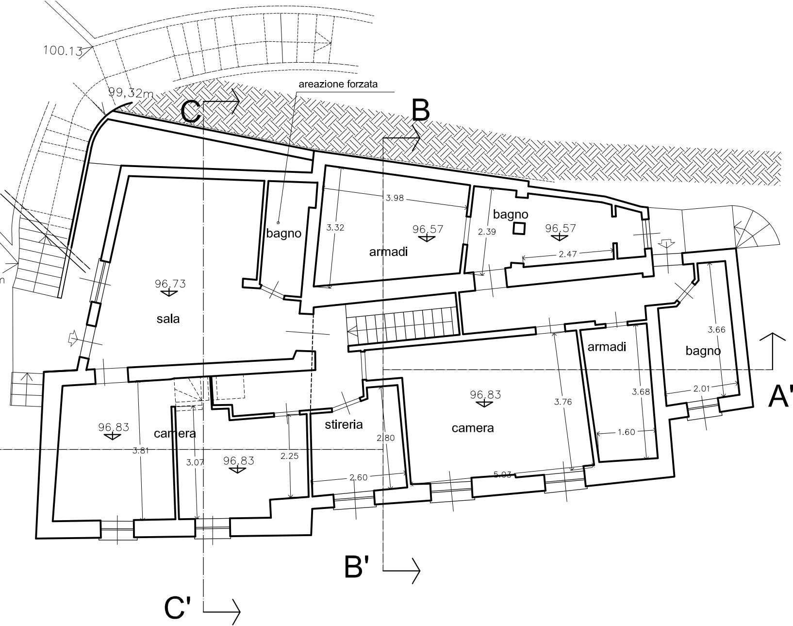
PIANO PRIMO
