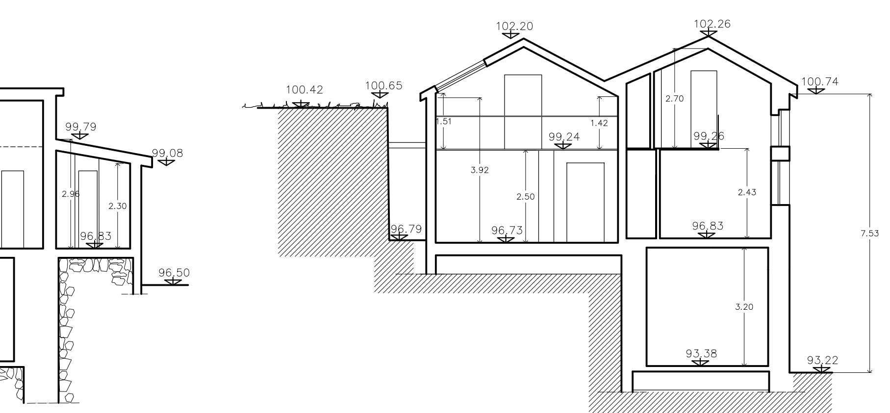
SEZIONE C-C'
