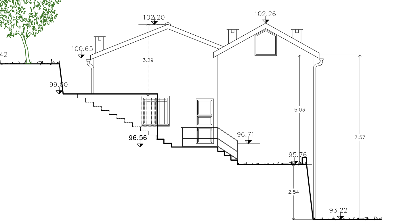
PROSPETTO NORD-OVEST
