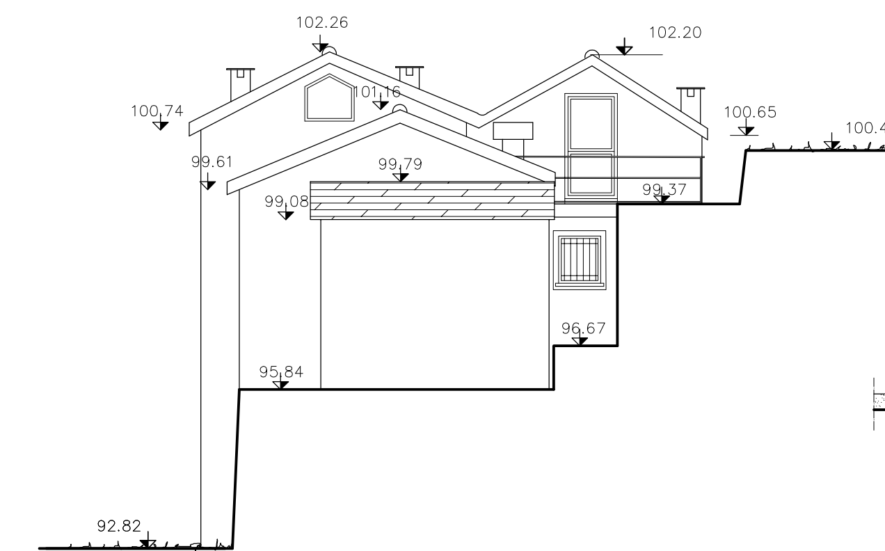
PROSPETTO SUD EST
