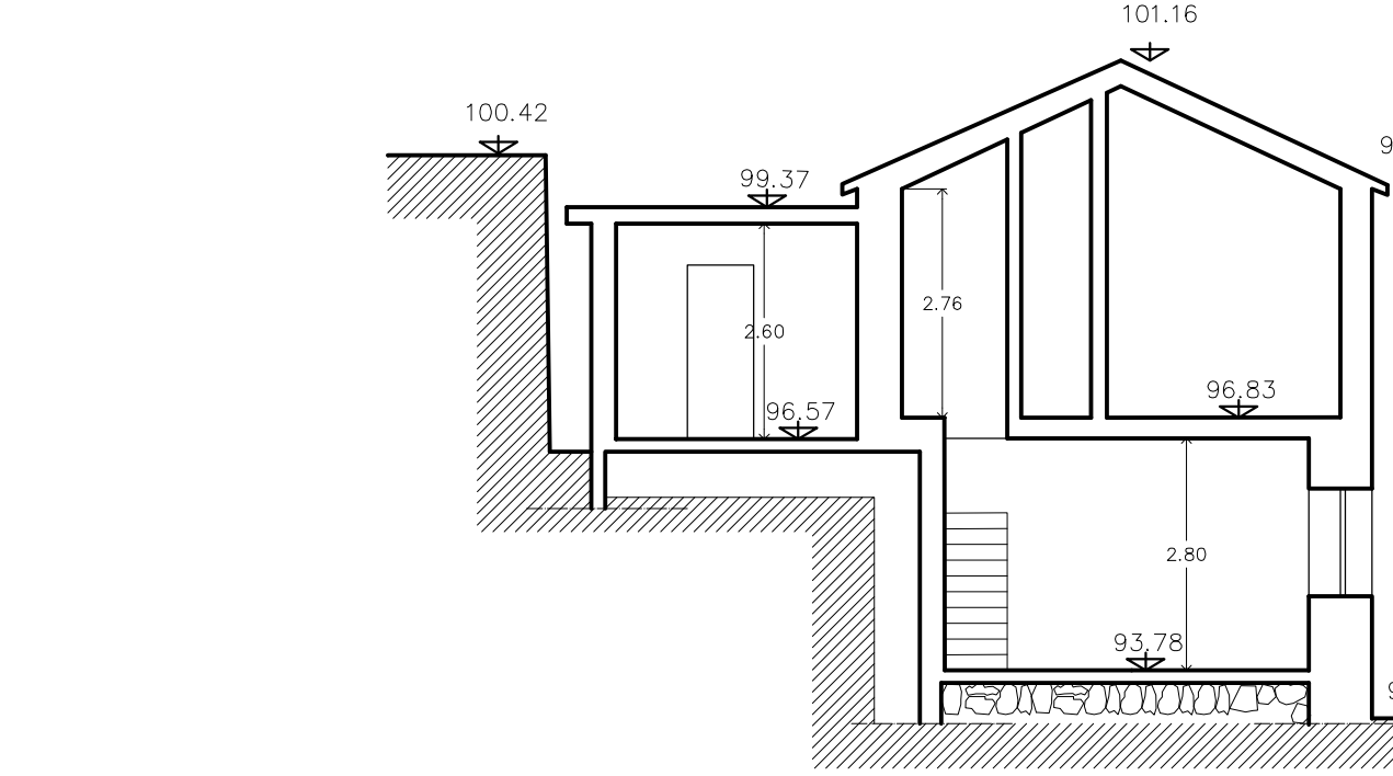
SEZIONE B-B'
