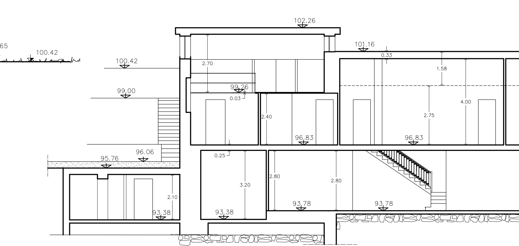
SEZIONE A-A'
