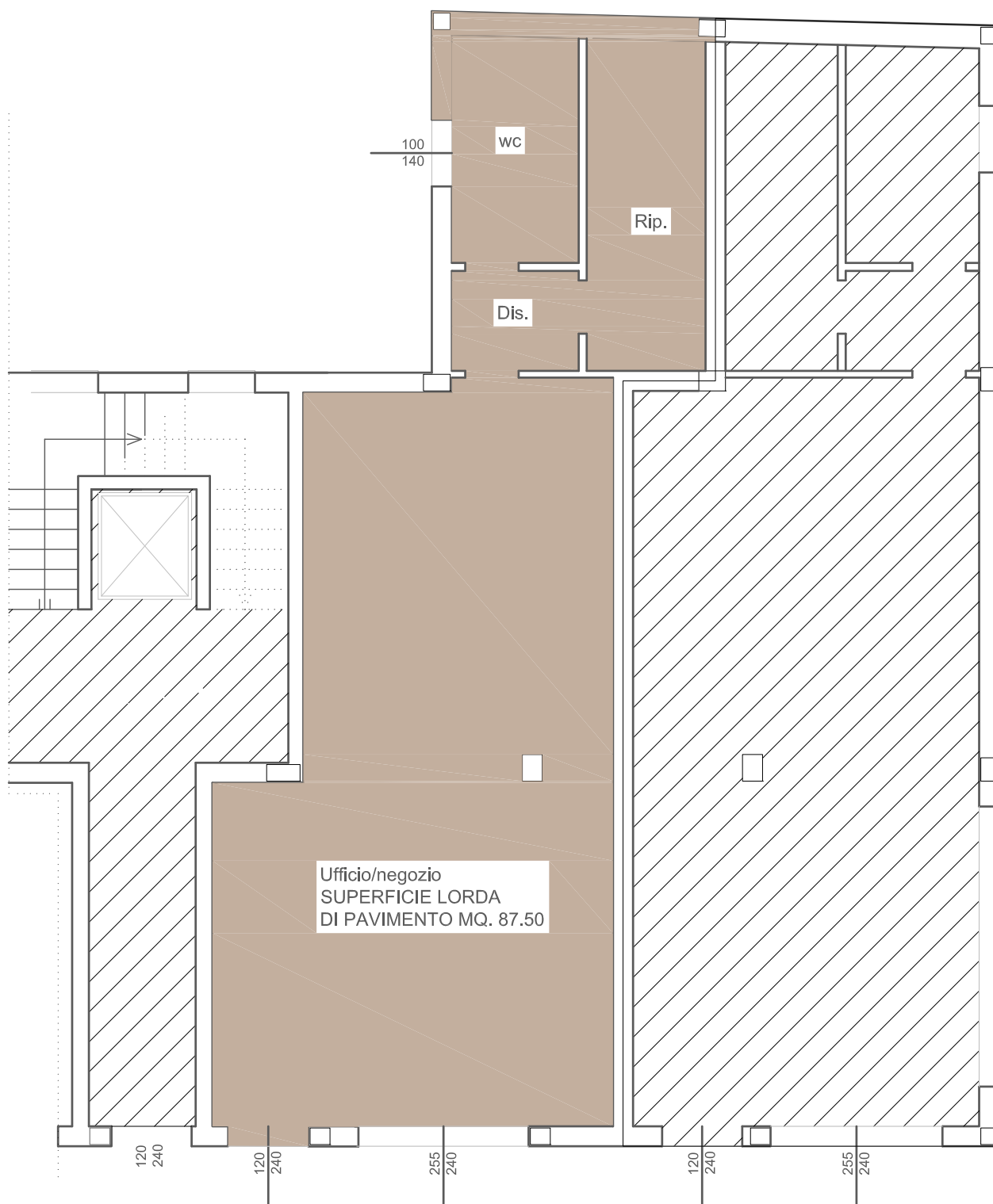
PIANTA PIANO TERRA SOLUZIONE COMMERCIALE
