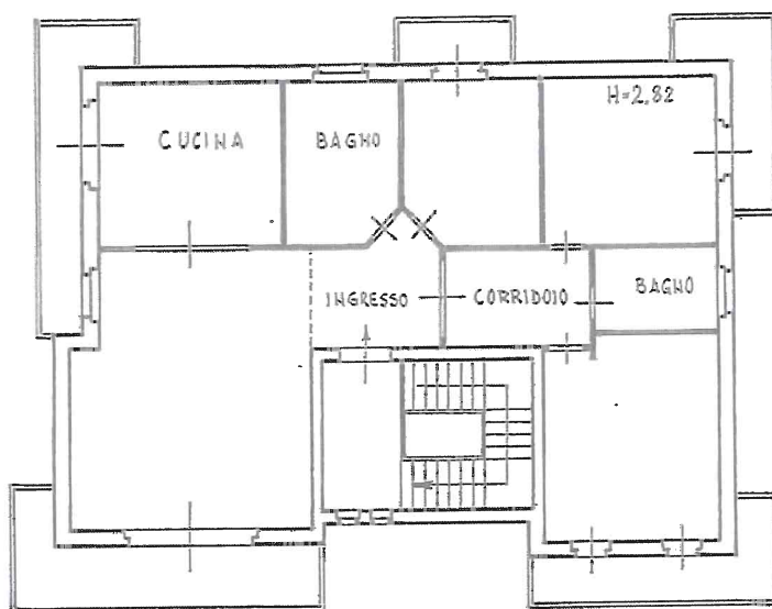
PIANO PRIMO
