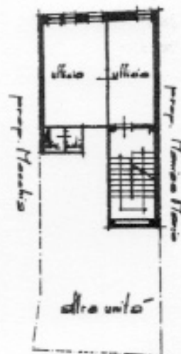
piano secondo H. 250
