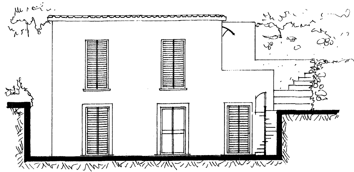
PROSPETTO C
