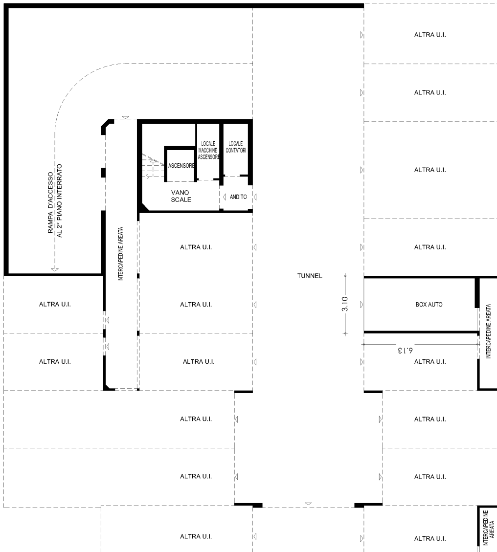
PIANO SECONDO INTERRATO - H : 2.64
